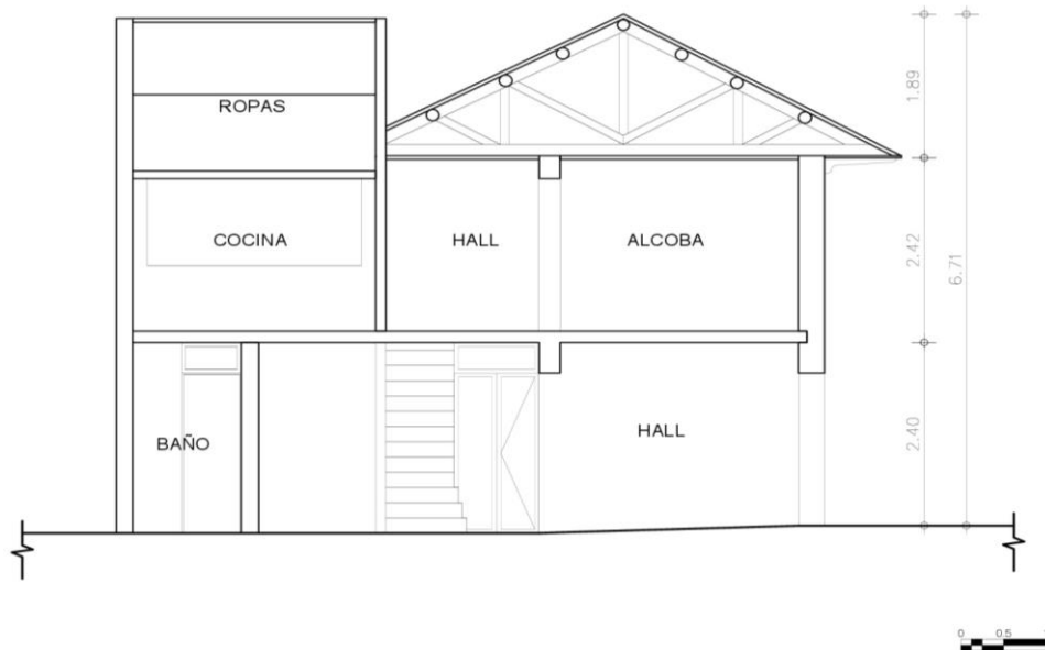
Corte longitudinal
